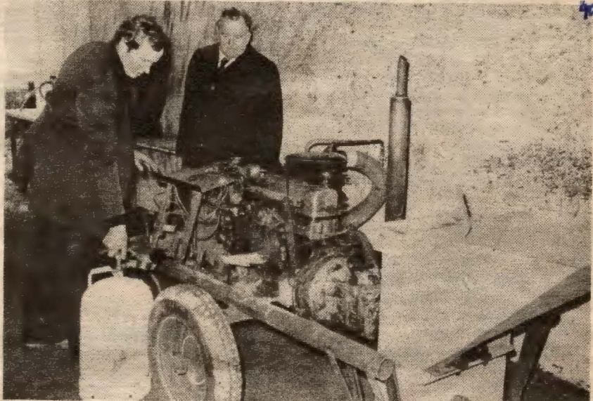
Josef Regl betreibt hier mit seinem Biogas-Pkw-Motor eine Zerkleinerungsmaschine (rechts Maschinenringgeschäftsführer Schachinger).
